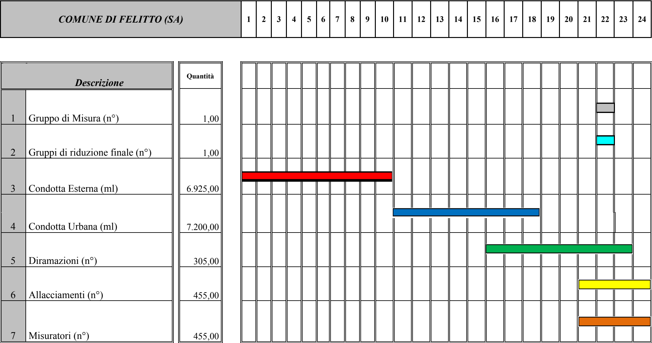
CRONOPROGRAMMA DEI LAVORI DI COSTRUZIONE IMPIANTO DI DISTRIBUZIONE GAS METANO (espresso in mesi)
